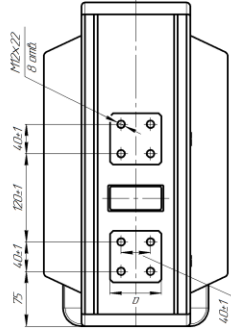
Рисунок А.3 — Габаритные, установочные, присоединительные размеры трансформаторов ТОЛ-НТЗ-35-11, -12
