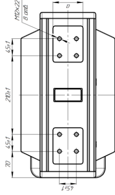
Рисунок А.3 — Габаритные, установочные, присоединительные размеры трансформаторов ТОЛ-НТЗ-35-11, -12
